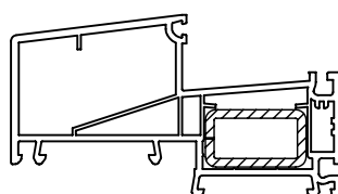
Армирование 35 x 20
