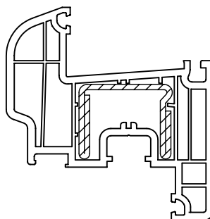
Армирование 35 x 28
