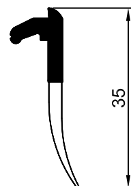
Арт. 553370 01 Нащельник 4
