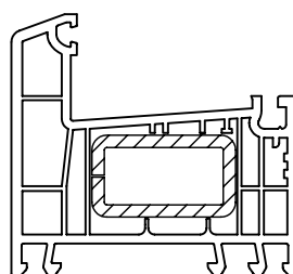
Армирование 35 x 20
