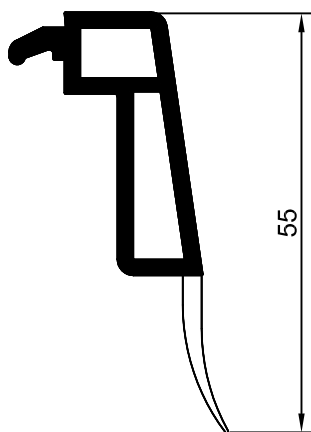
Арт. 553220 01 Нащельник 3
