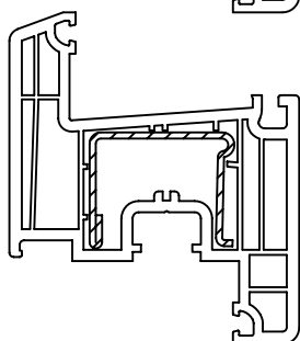
Армирование 35 x 28
