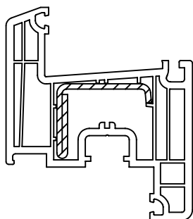
Армирование 35,5 x 28
