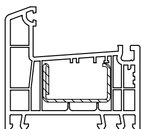
Армирование 35 x 20
