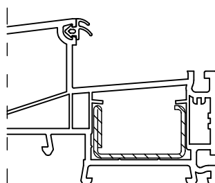
Уплотнитель притвора
