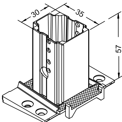
Арт. 221664 серебристый, хромированный цинкованный, литой Механический соединитель с уплотняющей подушкой для Импоста 86 BriD (M 1:2) Норма упаковки: 50 штук
