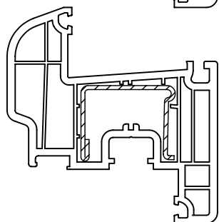
Армирование 35 x 28
