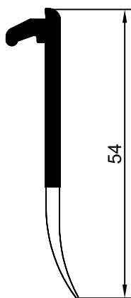
Арт. 553190 01 Нащельник 2
