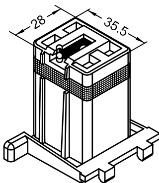
Арт. 247446 белый, коричневый, бежевый, карамель RAU-PA + 30% стекловолокно Механический соединитель с уплотняющей подушкой для Импоста 86 BriD (M 1:2) Норма упаковки: 90 штук
