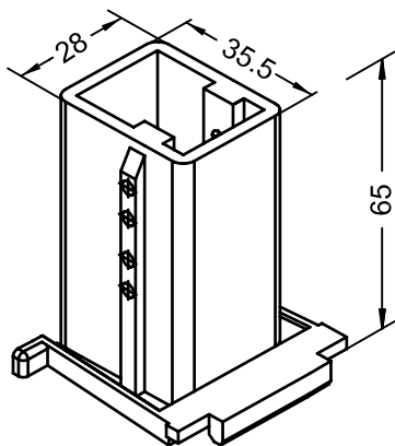
Арт. 242487 белый, коричневый, бежевый, карамель RAU-PA + 30% стекловолокно Механический соединитель с уплотняющим кольцом для Импоста 86 BriD (M 1:2) Норма упаковки: 60 штук
