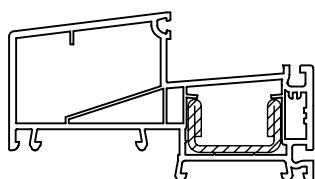
Армирование 35 x 20
