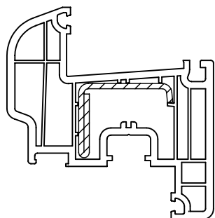
Армирование 35,5 x 28
