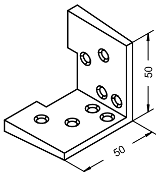
Арт. 226253 серебристый хромированный цинкованный, литой Монтажный уголок для горбылька 68 BriDi Импоста 86 BriD (M 1:2.5) (использование как светоделящего элемента в створке) Норма упаковки: 50 штук
