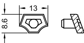
Арт. 241937 чёрный RAU-ABS Фиксатор Норма упаковки: 500 штук
