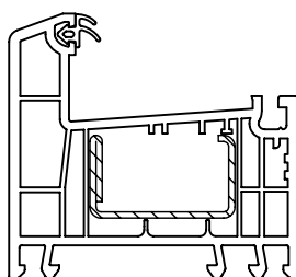
Уплотнитель притвора
