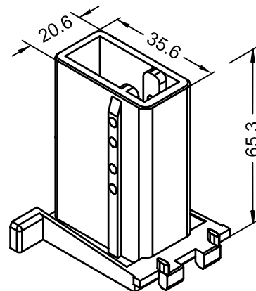
Арт. 229960 белый RAU-PA + 30% стекловолокно Механический соединитель с уплотняющим кольцом для импоста 78 Euro 70 (M 1:2) Норма упаковки: 100 штук
