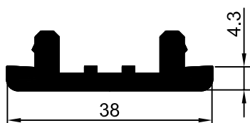
Арт. 553210 01 Соединительный профиль
